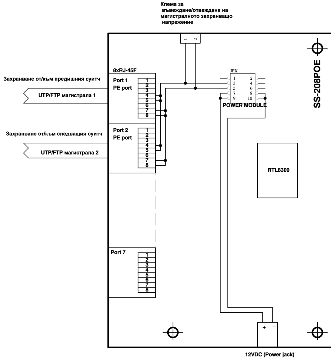
Принципна схема на SmartSwitch с PoE връзките
